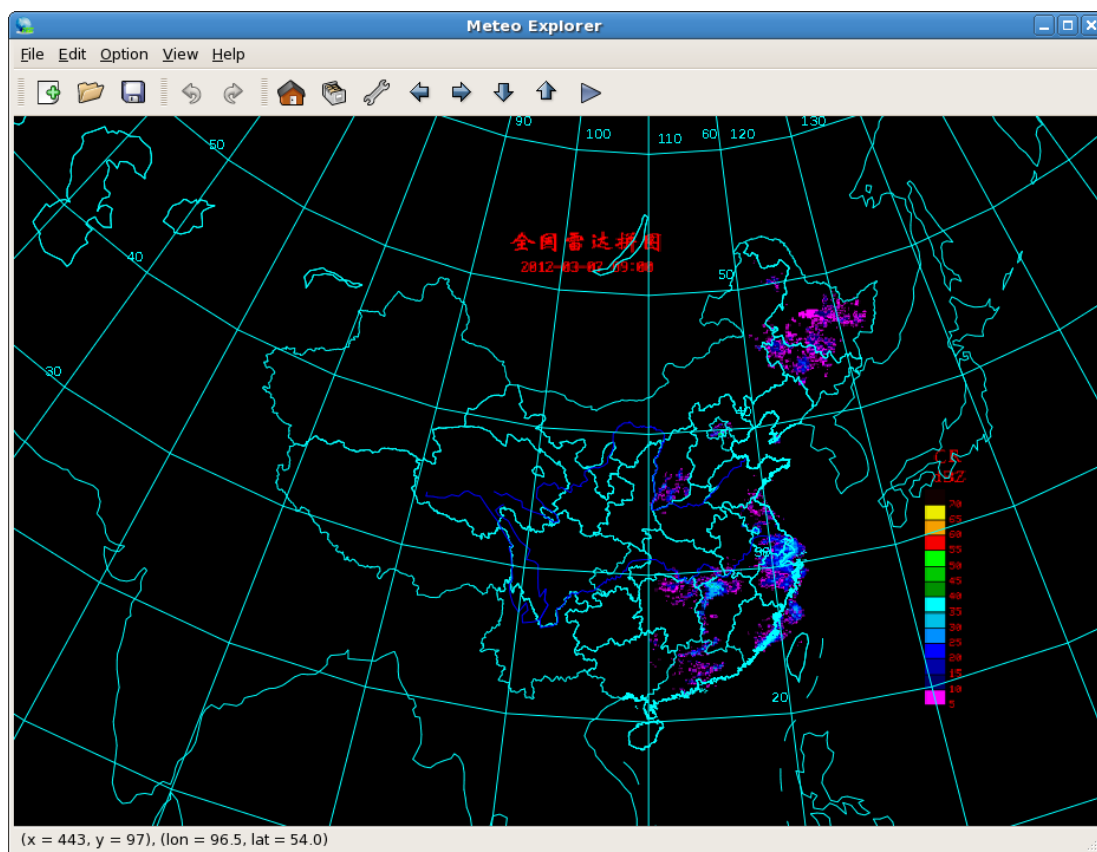
图 15-5: MeteoExplorer 中显示的全国雷达拼图图像。
