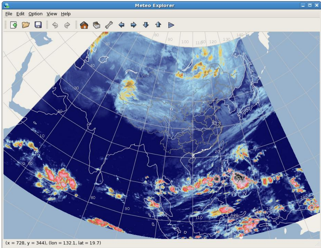
图 15-2: 风云二号卫星拍摄的一幅 AWX 格式的红外云图图像显示结果。
