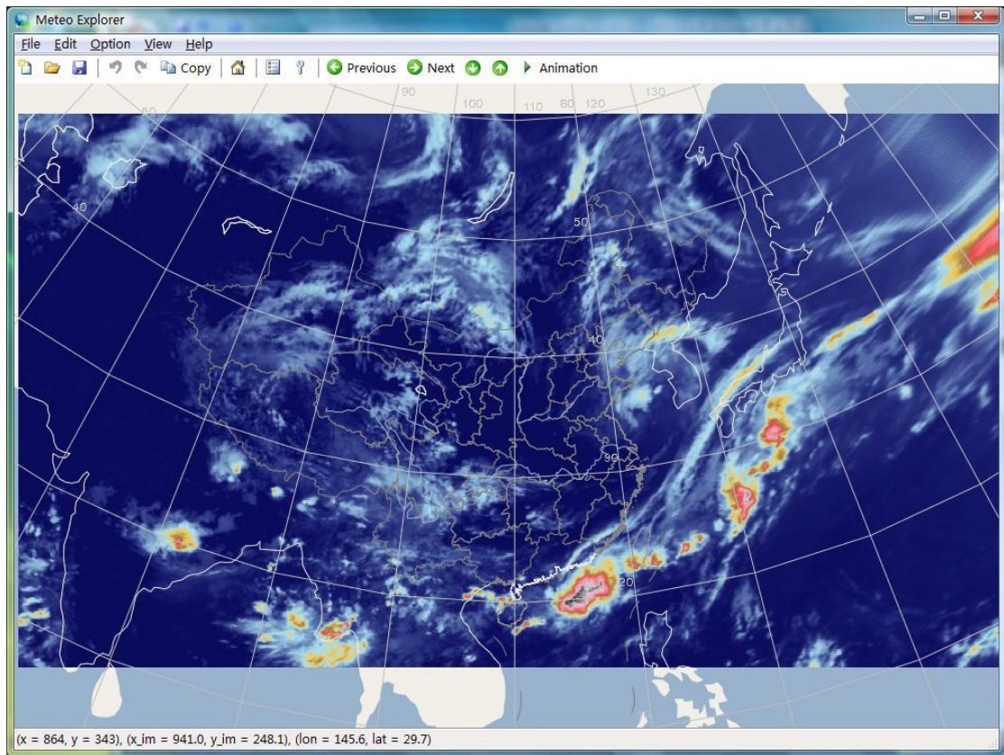
图 15-6: MeteoExplorer 中显示的 GPF 格式的高分辨率多通道云图。
