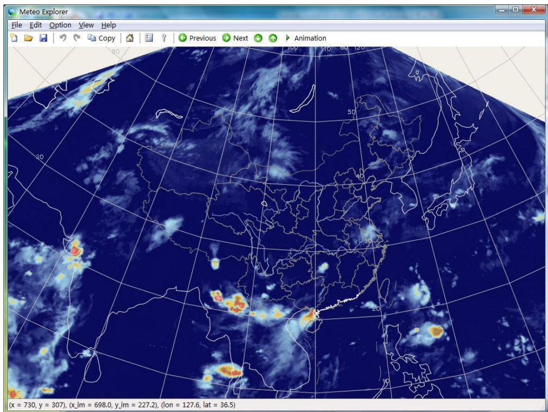
图 15-7: MeteoExplorer 中显示的 HDF 格式的高分辨率多通道云图。
