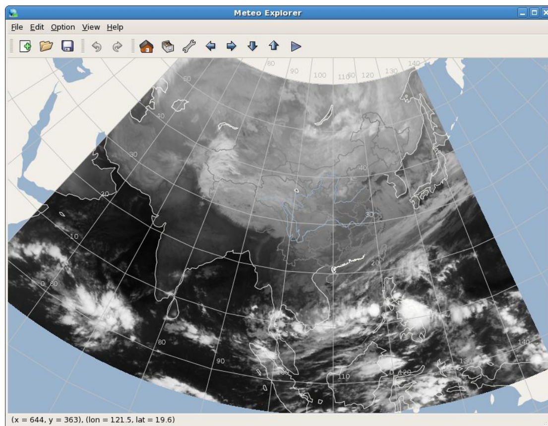
图 15-4: 图 15-2 中红外云图图像在灰度级别调色板下的显示结果。
